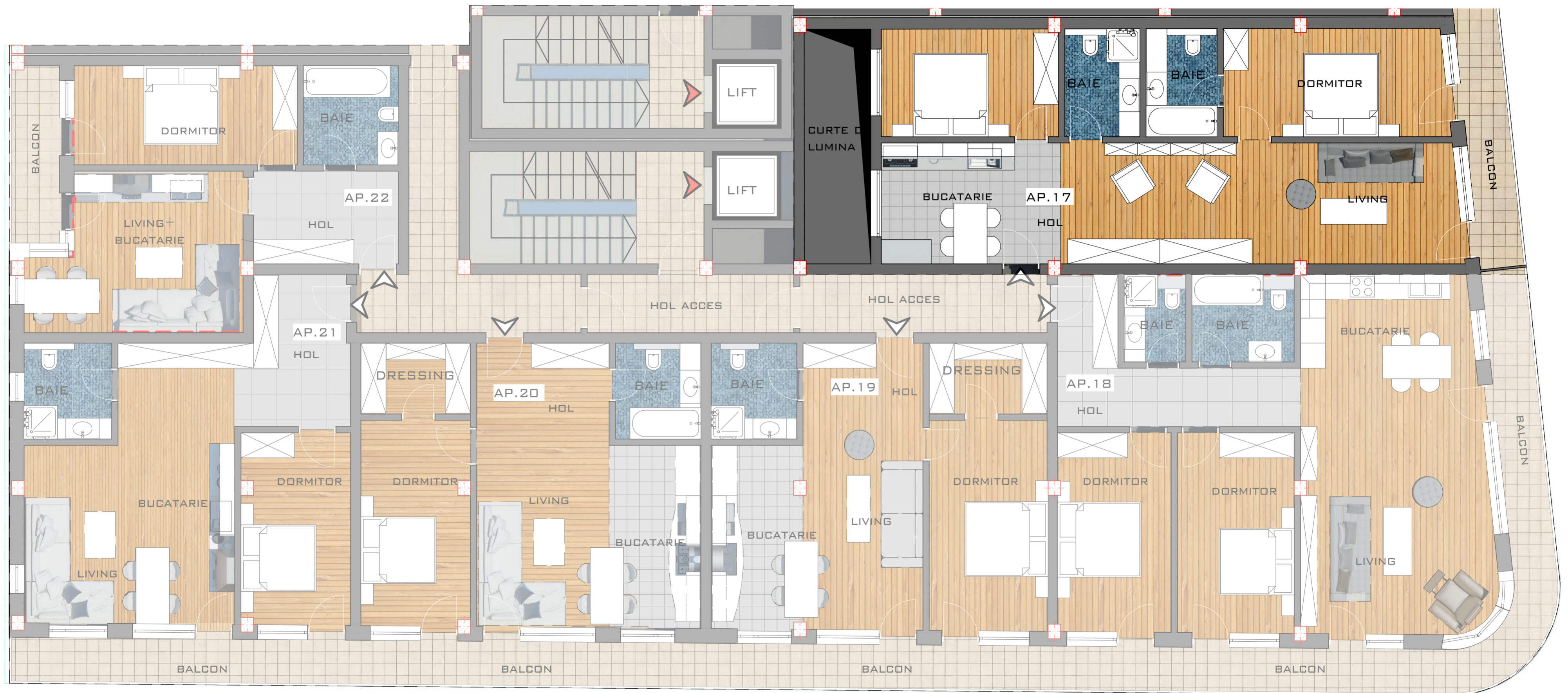
PLAN ETAJ 12
